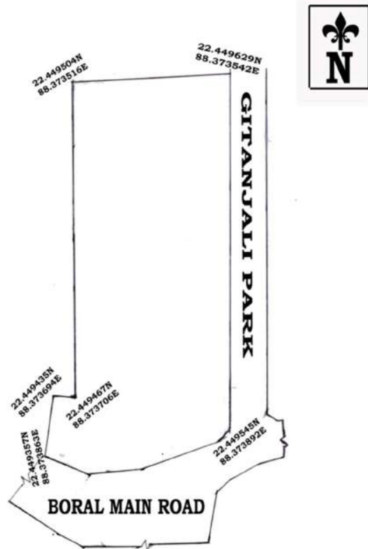
SITE PLAN WITH LATITUDE LONGITUDE
